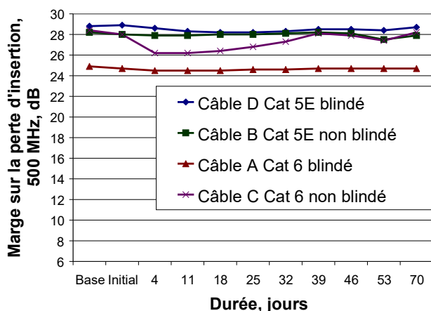
Câbles de données insérés dans un conduit fermé de 30 m
